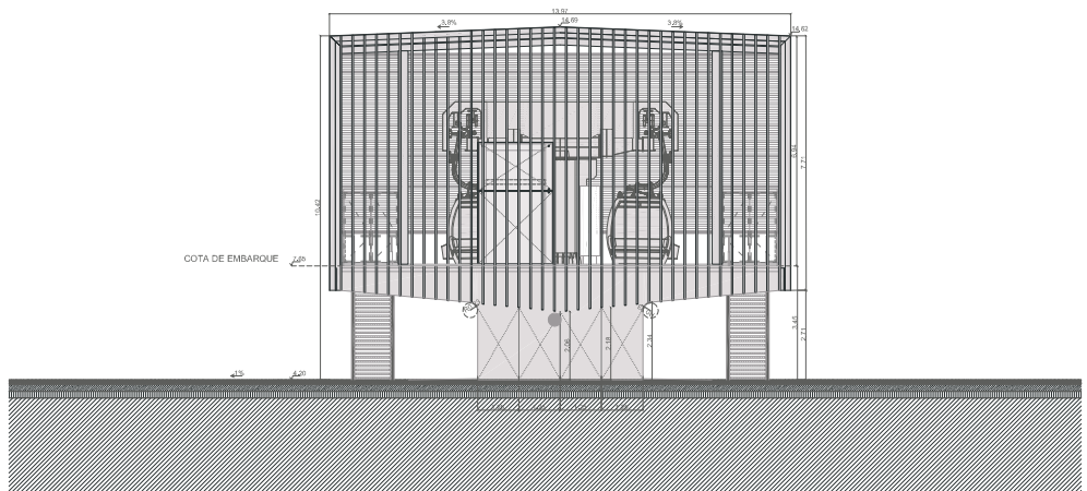
alçado poente
