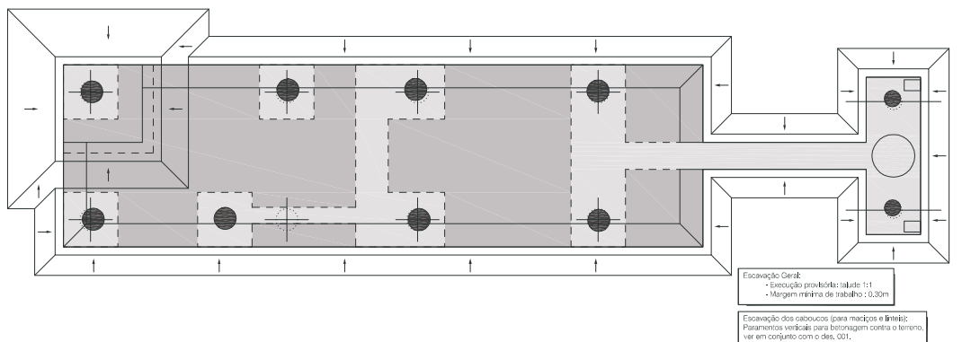
planta - zona de abertura de caboucos para fundações
