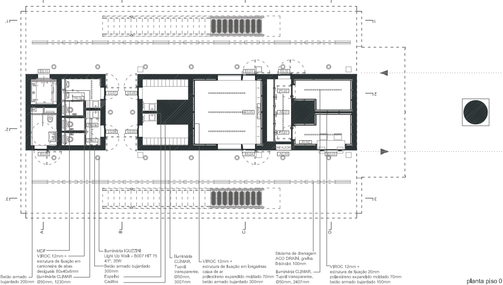
planta piso 0
