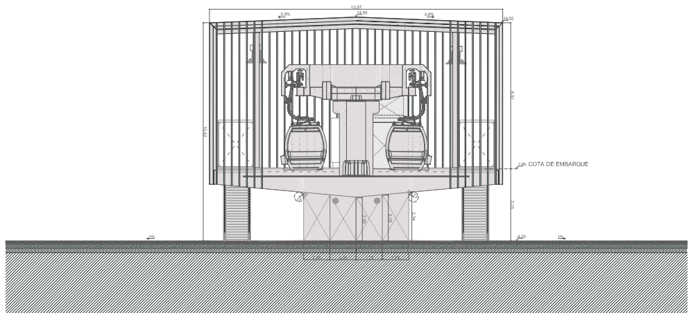
alçado nascente
