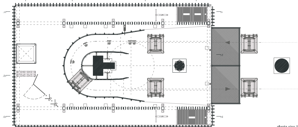
planta piso 1
