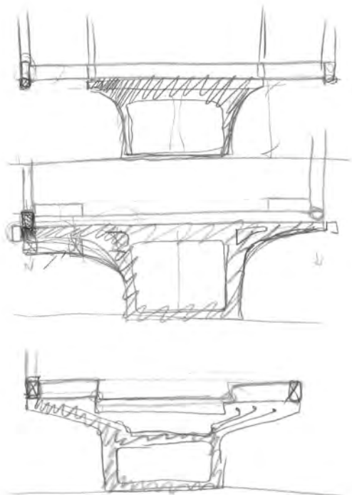
esquisso da consola e estrutura metálica
