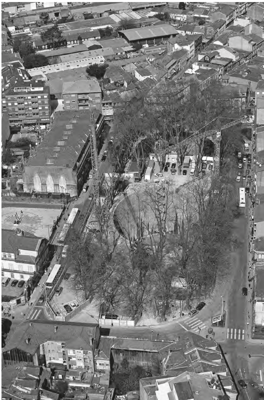
Estação Marquês - parte central escavada em poço, foto aérea
