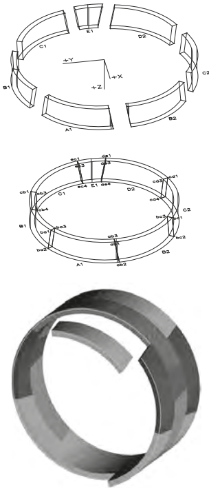
Aduelas de um anel Imagem gerada pelo software de escolha de posição dos anéis para o traçado pretendido – ordem de montagem
