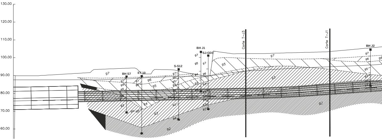
Planta do túnel da Linha J Perfil longitudinal do túnel da Linha J com indicação das várias unidades geotécnicas
