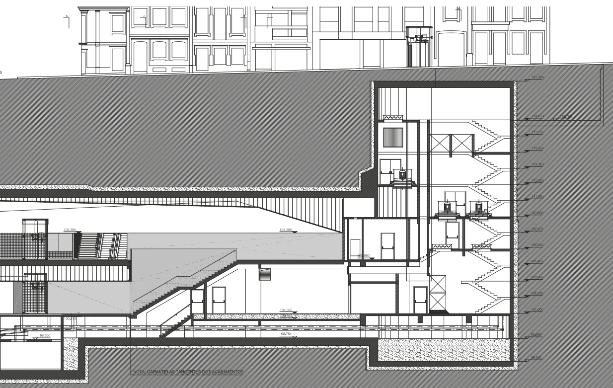
Corte transversal da estação Faria Guimarães
