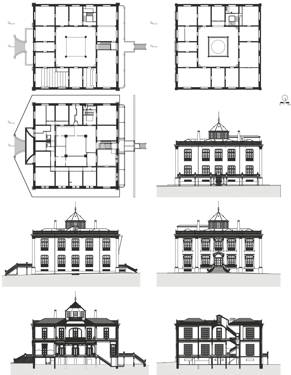
Fig. 6. Desenhos de levantamento: plantas do rés-do-chão, 1.º andar e cave; alçados sul, poente e da rua do Campo Alegre; cortes longitudinais CL1 e CL2.
