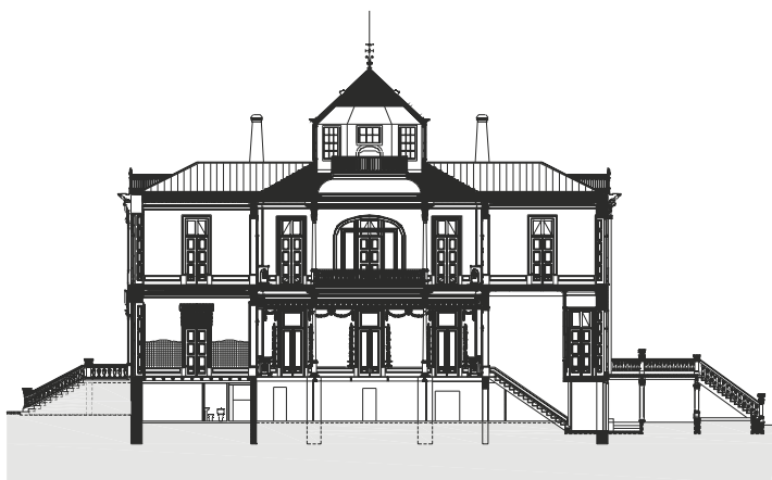
Fig. 10. Desenhos da proposta Corte Longitudinal CL2 (1.ª fase) Corte Longitudinal CL1 (1.ª fase).
