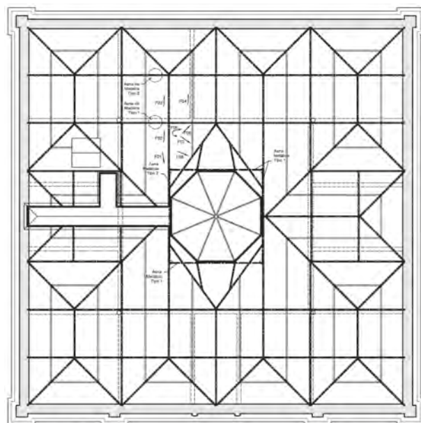
Planta Estrutural de Cobertura (Tecto do Piso 3)
