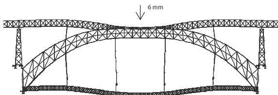
Malha deformada para o caso de carga 2.
