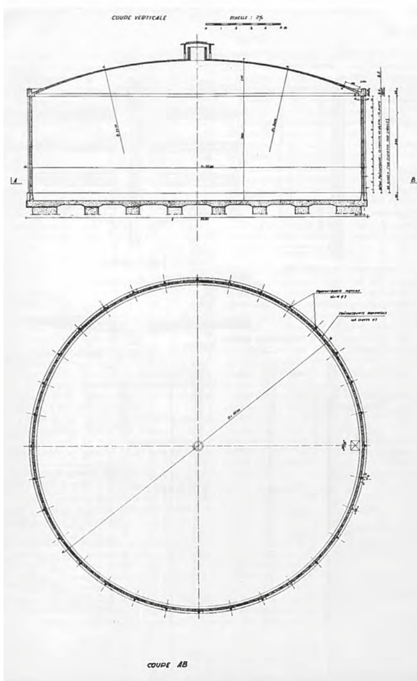
Transferência de água entre o Depósito de Santo Isidro e o Depósito dos Congregados. Depósito principal, planta e corte vertical, in Sarmento, Eng. Albano Rodrigues do Carmo, Notícia sobre o Novo Depósito dos Congregados , na cidade do Porto, Instituto Superior Técnico, Lisboa, 1958.
