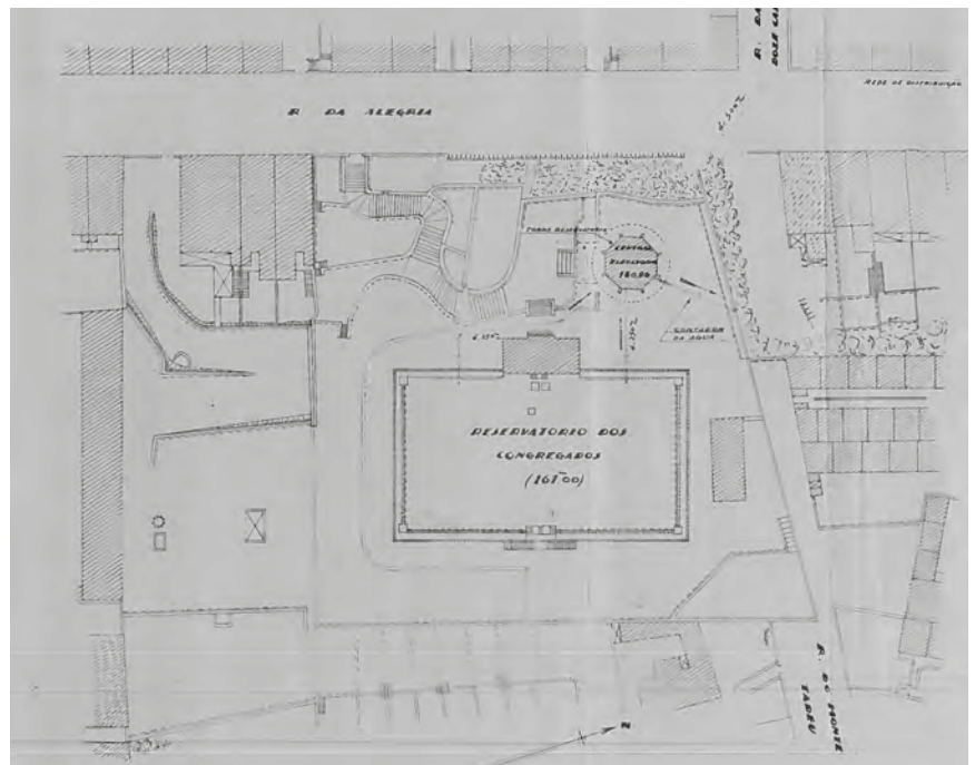
Transferência de água entre o Depósito de Santo Isidro e o Depósito dos Congregados. Esquema de distribuição, planta de localização e corte esquemático, in Sarmento, Eng. Albano Rodrigues do Carmo, Notícia sobre o Novo Depósito dos Congregados , na cidade do Porto, Instituto Superior Técnico, Lisboa, 1958.
