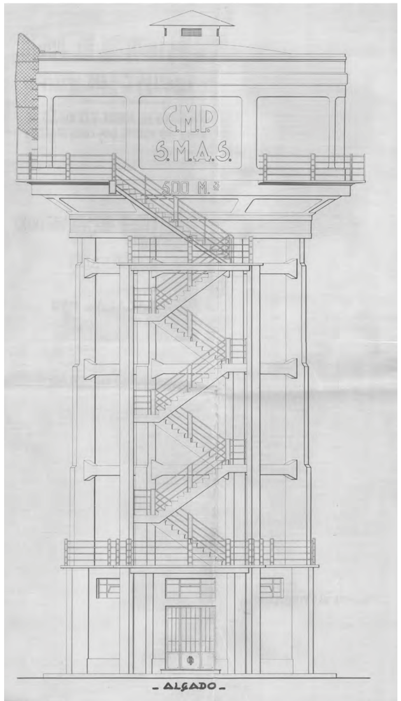
Torre de Pressão do Reservatório dos Congregados, alçado principal, 1937
