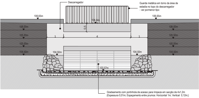
Vista Frontal a Montante
