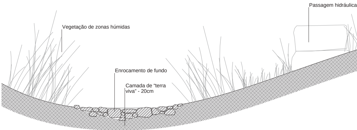
Pormenor tipo de bacias de retenção - planta e corte transversal
