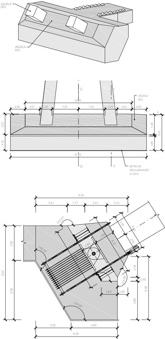
Fig. 26. Fundações das escoras
