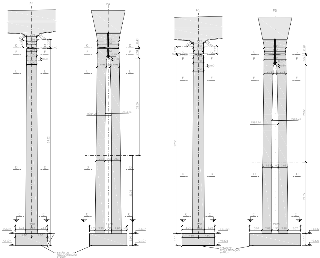
Fig. 27. Pilares P4 e P5
