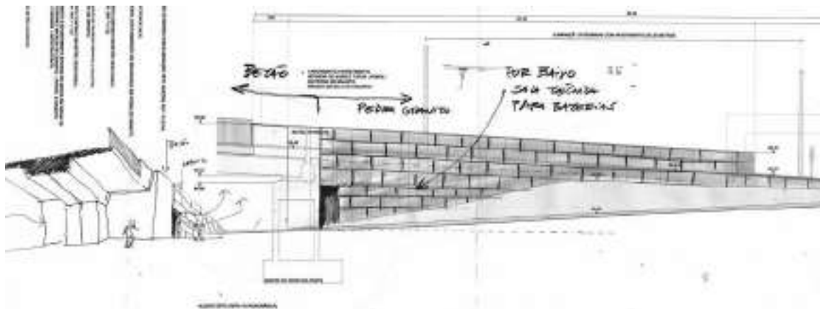
Fig. 32 e 33. Esquissos – estudos das estruturas do encontro da ponte, FAUP, Porto
