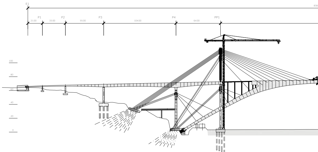
Fig. 29. Procedimento de construção
