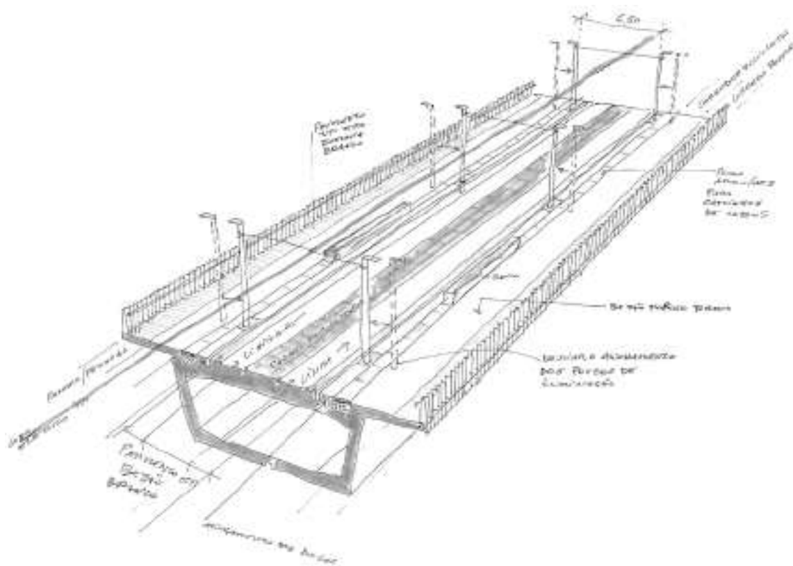
Fig. 18. Esquisso - axonometria
