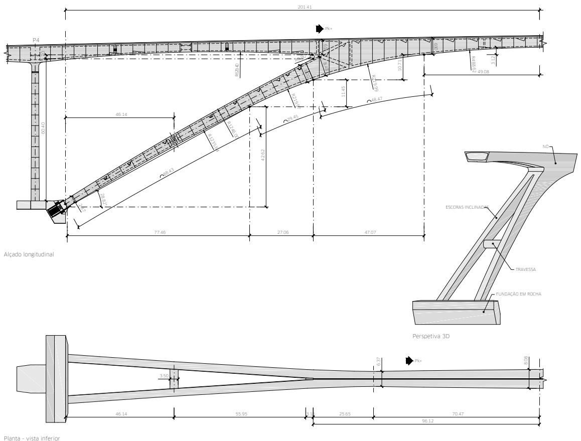
Fig. 28. Escoras inclinadas
