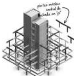
Fase 4: Elevação do Aço da Fachada Central
