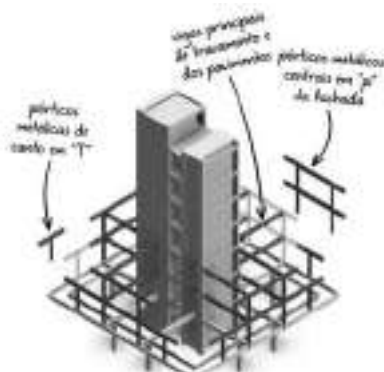
Fase 2: Elevação do Aço Central e Inferior da Fachada
