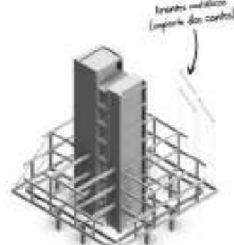
Fase 3: Montagem dos Tirantes de Suporte dos Cantos
