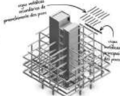
Fase 6: Instalação das Vigas Secundárias e Lajes
